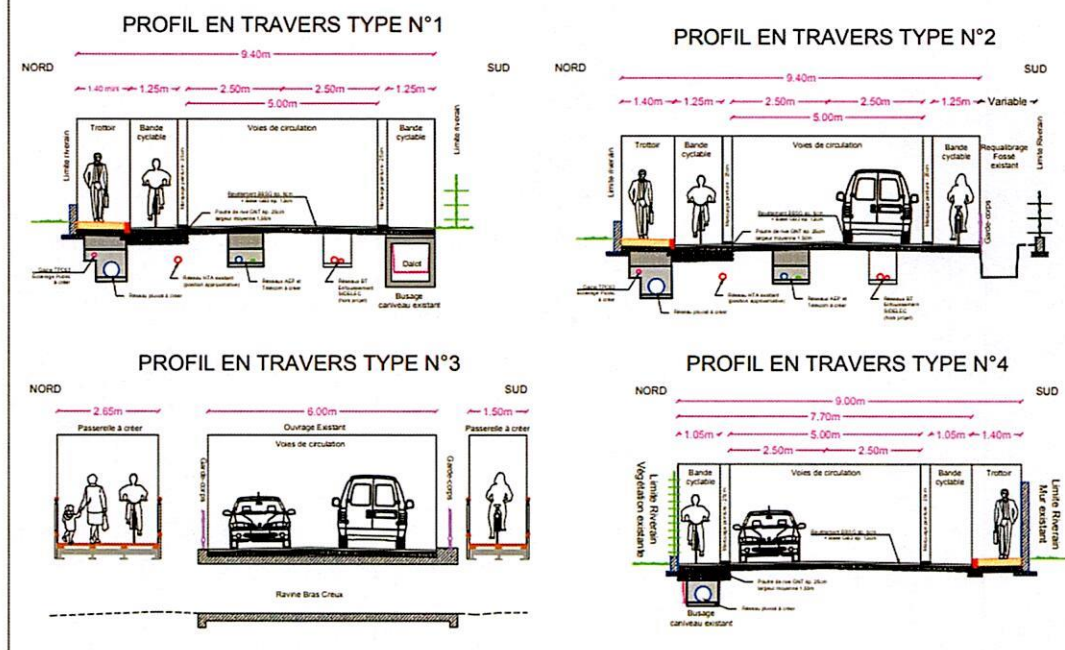
Profils type en travers
